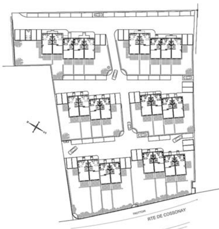
Plan masse
