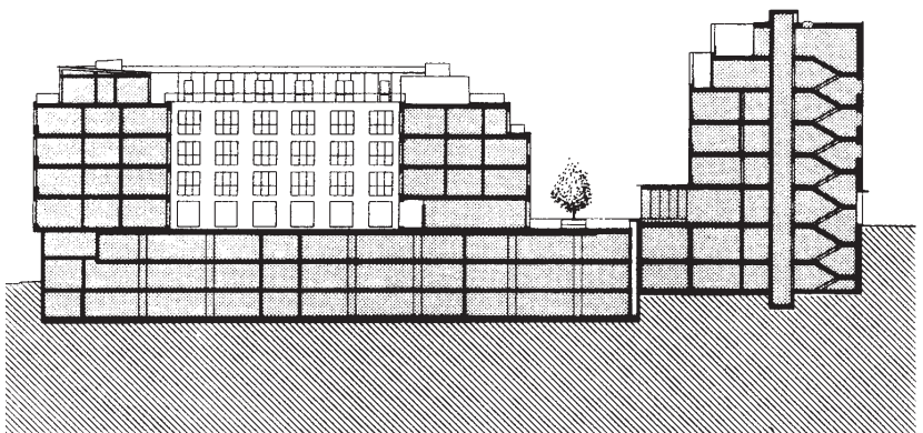
Coupe N-S
