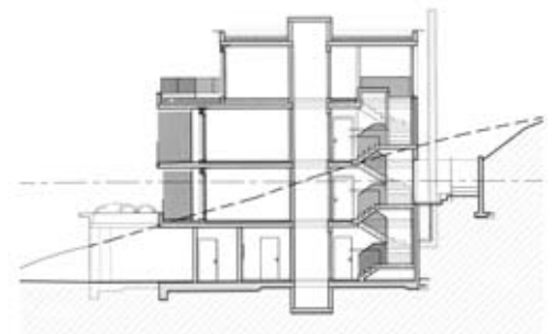
Coupe transversale
