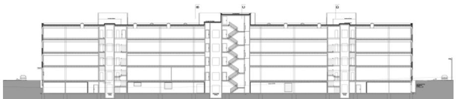
Coupe longitudinale
